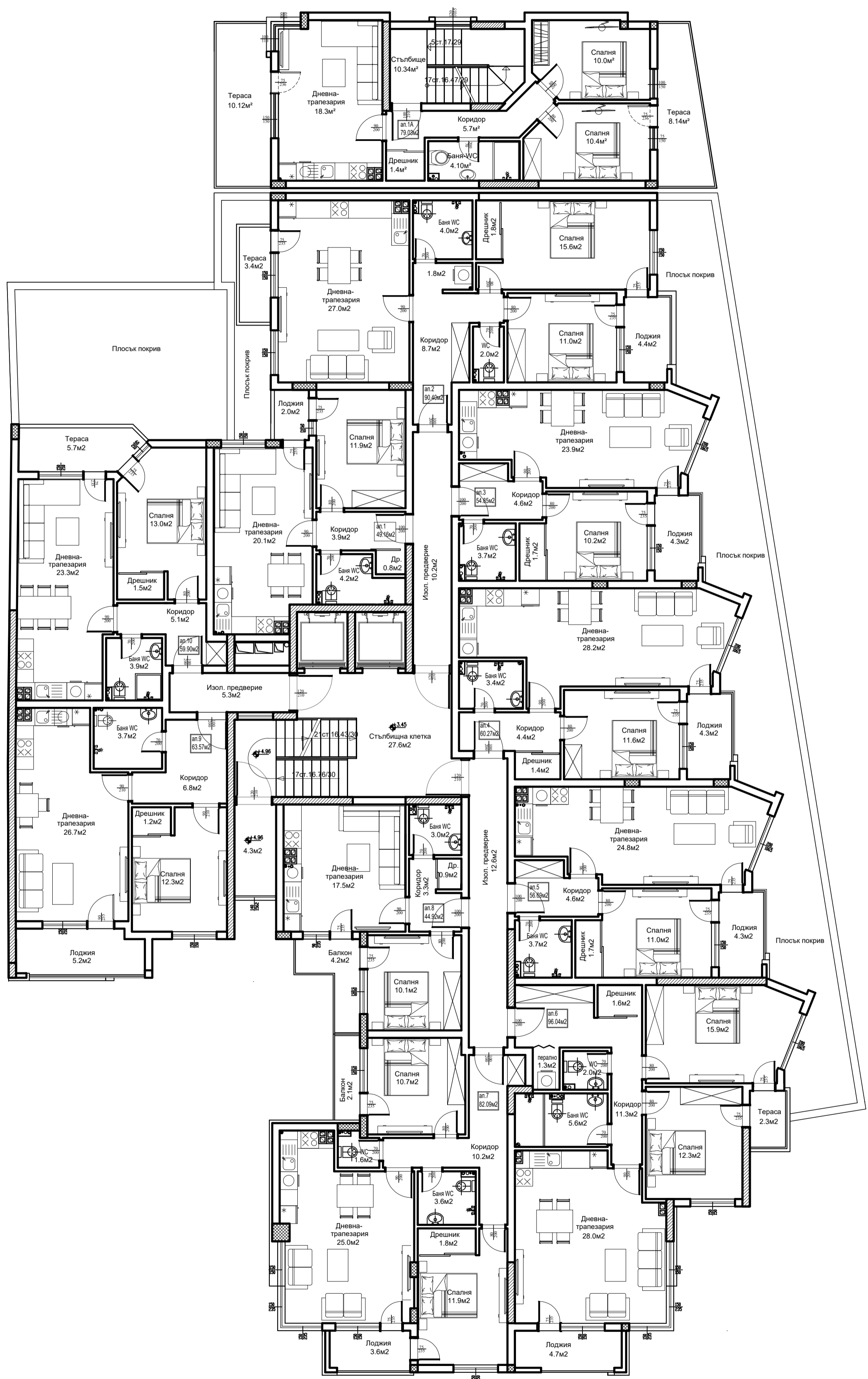
РАЗПРЕДЕЛЕНИЕ ВТОРИ ЕТАЖ
